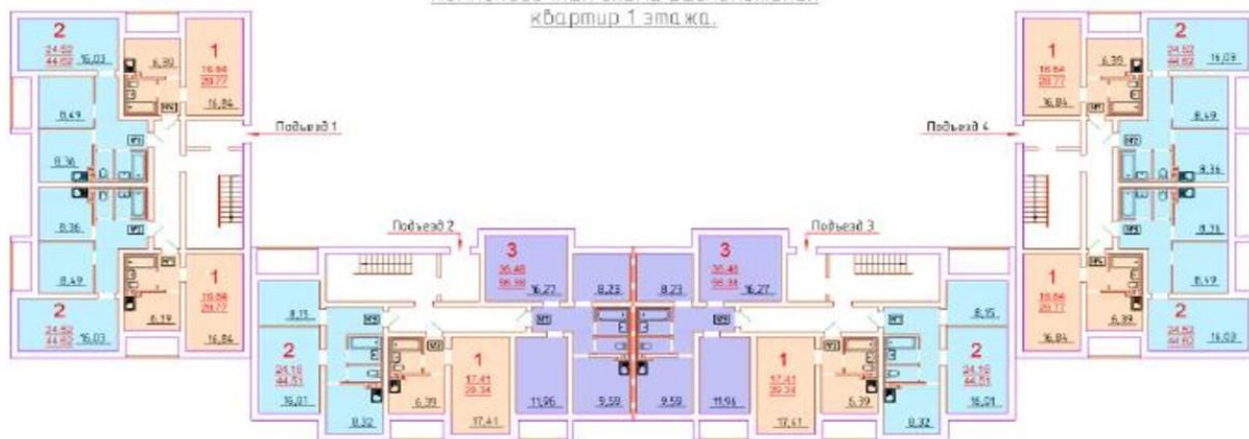
Компоновочная схема расположения квартир 1 этажа.
